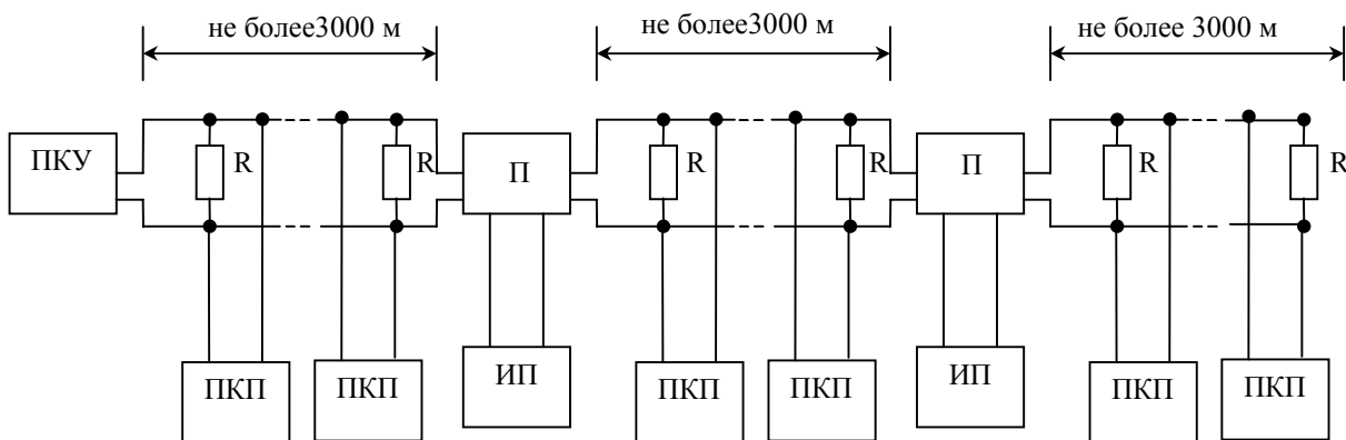
Рисунок 3 Увеличение длины линии с помощью повторителей интерфейса RS-485
